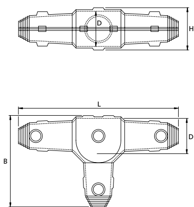
Dimensions T1
